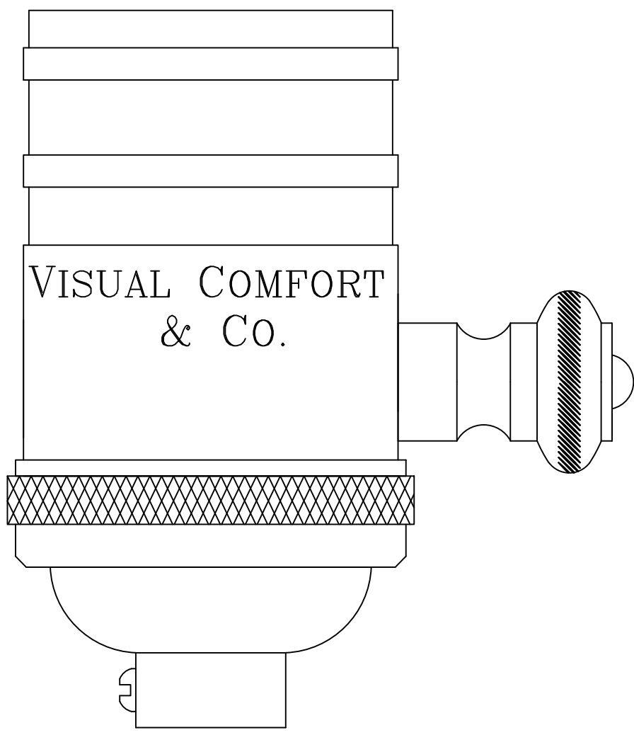
灯头左视图 SCALE 2:1
